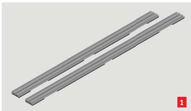
Grundprofil mit Bautenschutzmatte (gummibasiert oder alukaschiert) Länge 2370 oder 2490 mm
