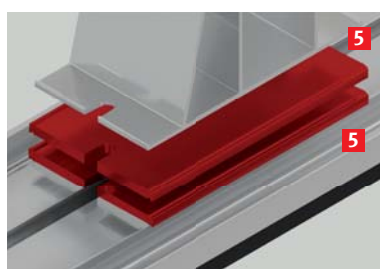
Höhenausgleich mit einer oder mehreren Stützenscheiben 5
