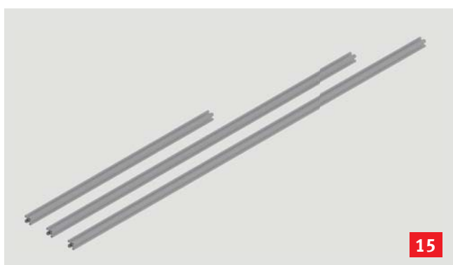
Montagehilfe-Profil 40 x 40 Standard für Modulbreite bis 1150 mm, Modullänge bis 1820 mm oder bis 2200 mm
