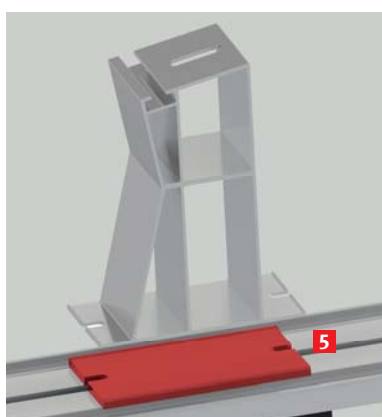
Höhenausgleich mit einer oder mehreren Stützenscheiben 5
