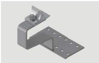
Einfacher Pfannenziegel-Dachhaken mit Schnelladapter
