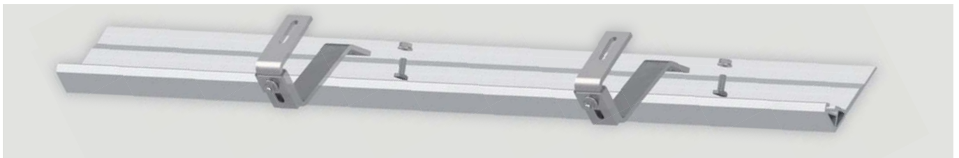
2-fach höhenverstellbarer Pfannenziegel-Dachhaken mit großer Fußplatte Geeignet für Dachrandbereiche und Dachhindernisse (zum Beispiel Schornstein oder Dachfenster)
