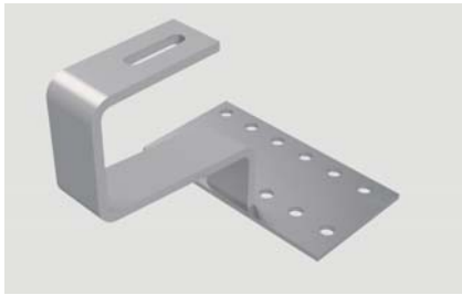
Einfacher Pfannenziegel-Dachhaken
