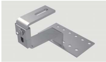
Höhenverstellbarer Pfannenziegel-Dachhaken
