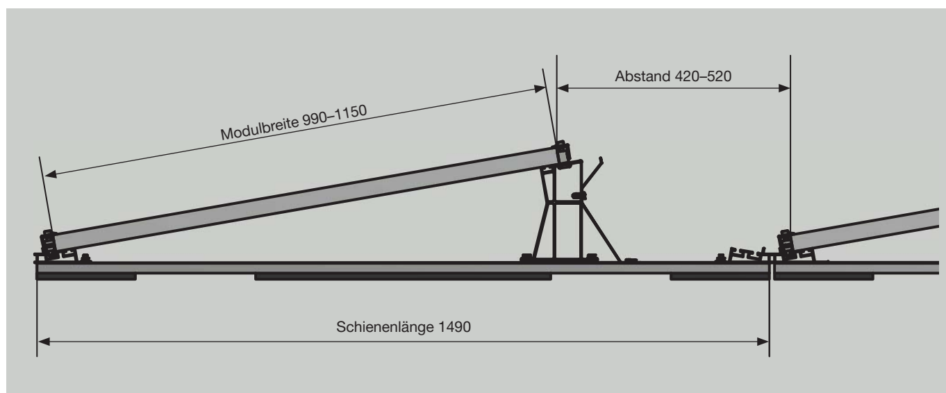
Beispiel Süd-System, Klemmung an der langen Seite
