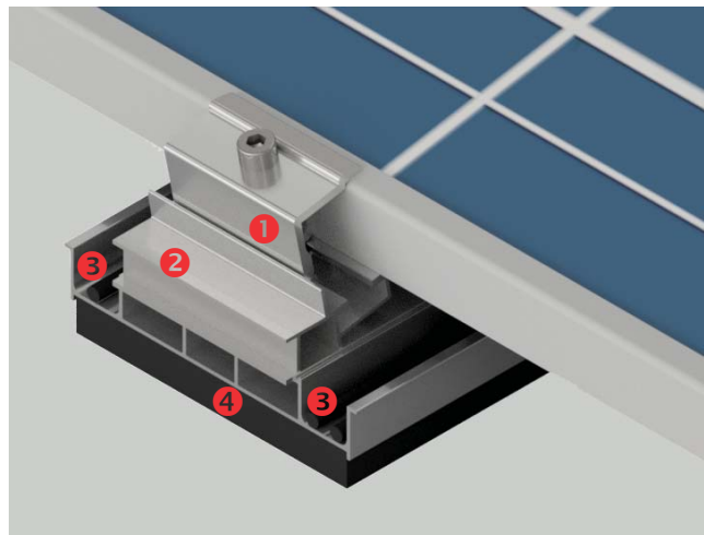
Klemmung an der langen Seite
