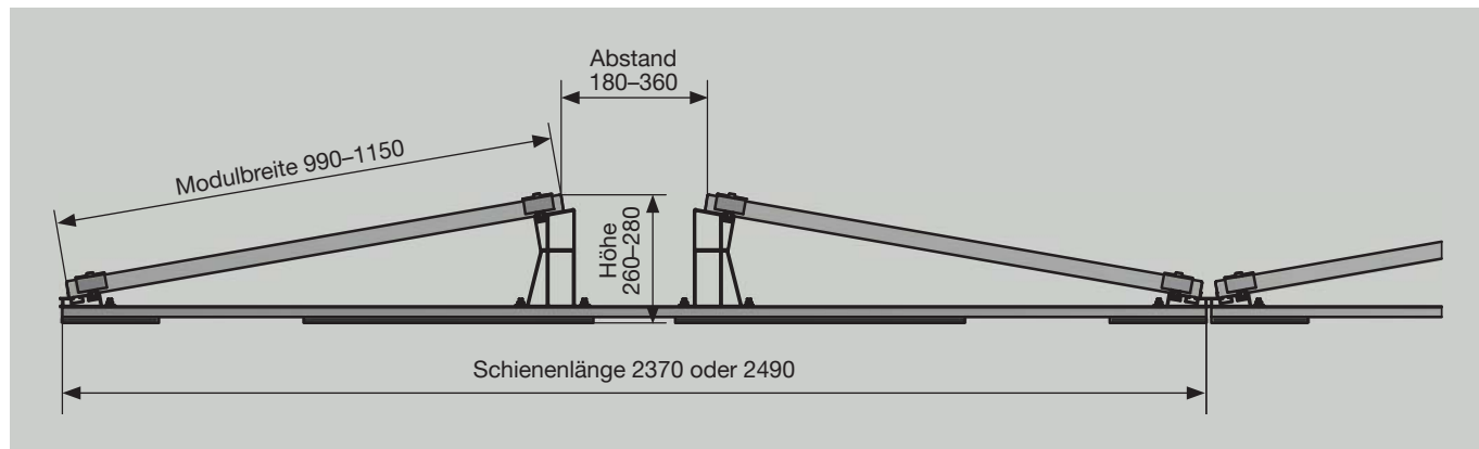
Beispiel Ost-West-System, Klemmung an der kurzen Seite
